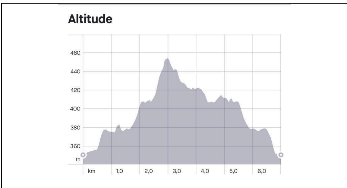
Figure B4 – Profil de dénivelé du parcours Rouge (7.0 km, 135 m +)
